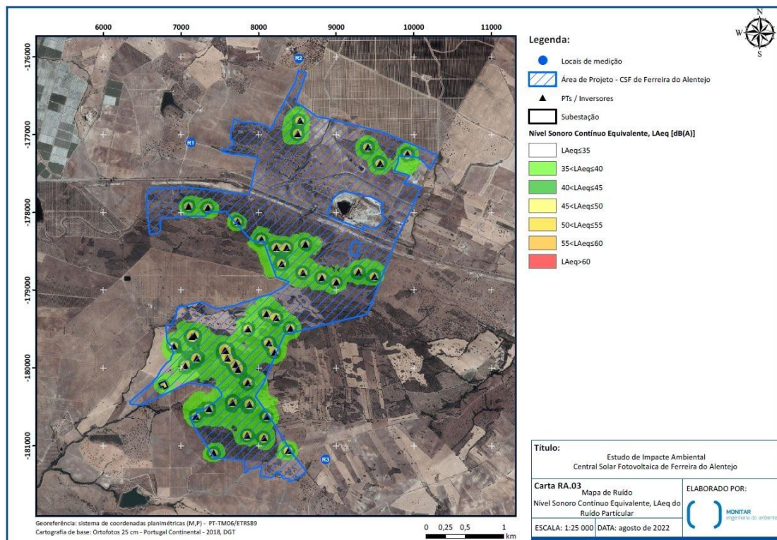
Figura 7: Mapa de ruído previsual associado ao funcionamento da CSF de Ferreira do Alentejo, na fase de exploração, para o indicador LAeq em período diurno. Fonte: adaptado do EIA, Anexo 5 do Volume 3, 2022.
