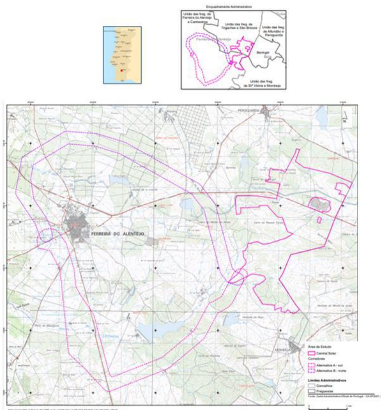
Figura 1 – Representação dos dois corredores de linha (A – a sul e B – a norte). (Fonte: Resumo Não Técnico)
